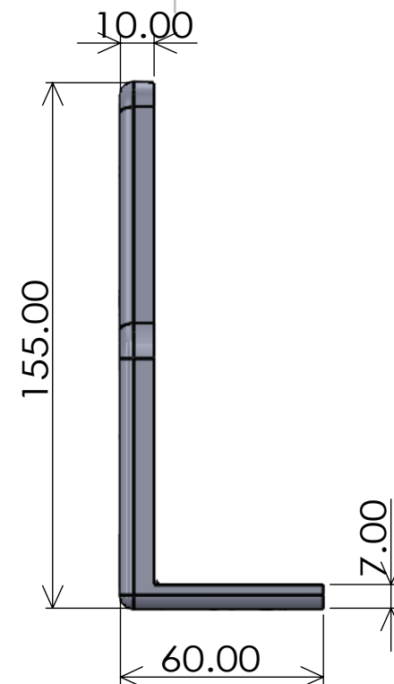
側面 スケール1/2
