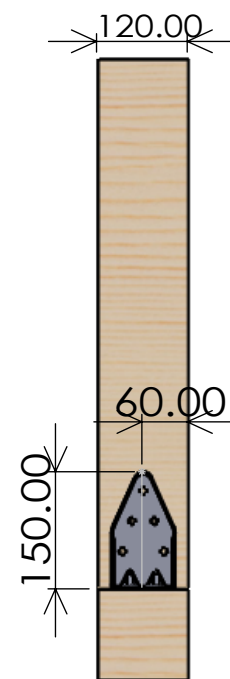
正面 スケール1/10
