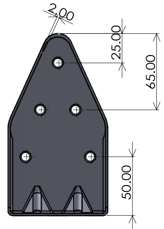
裏面 スケール1/2
