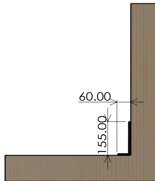
側面 スケール1/10
